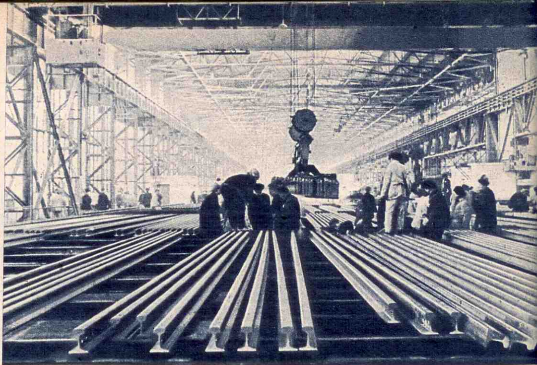
Рельсoproкатный цех Аньшаньского металлургического комбината.
